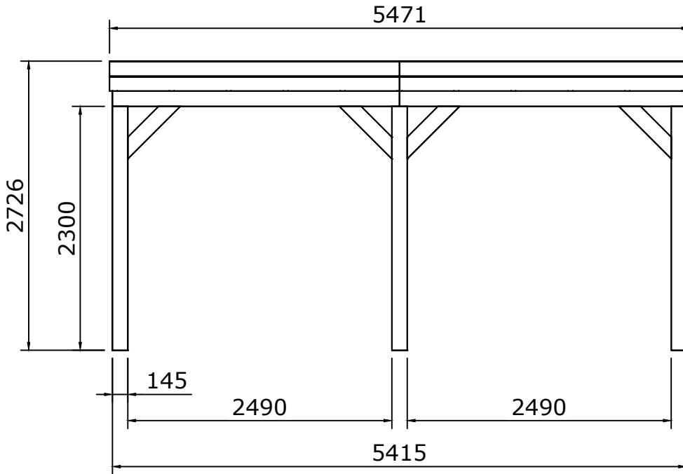
Vooraanzicht
