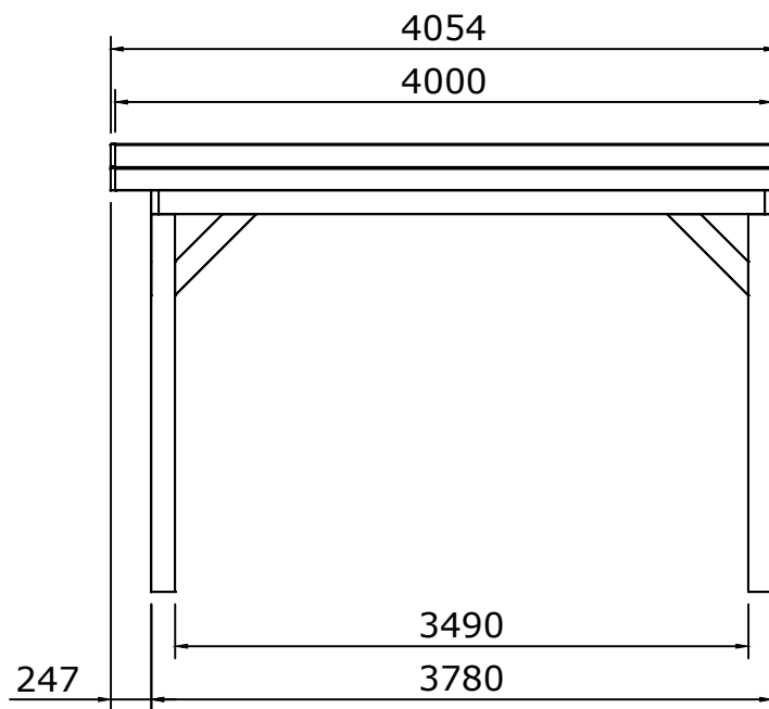
Rechter zijaanzicht
