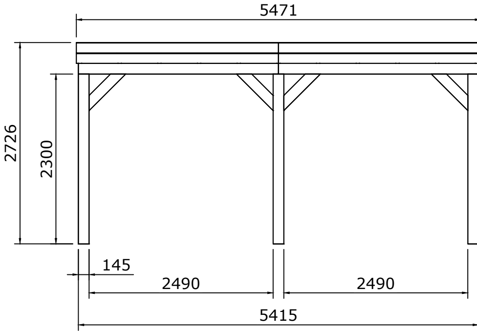
Vooraanzicht
