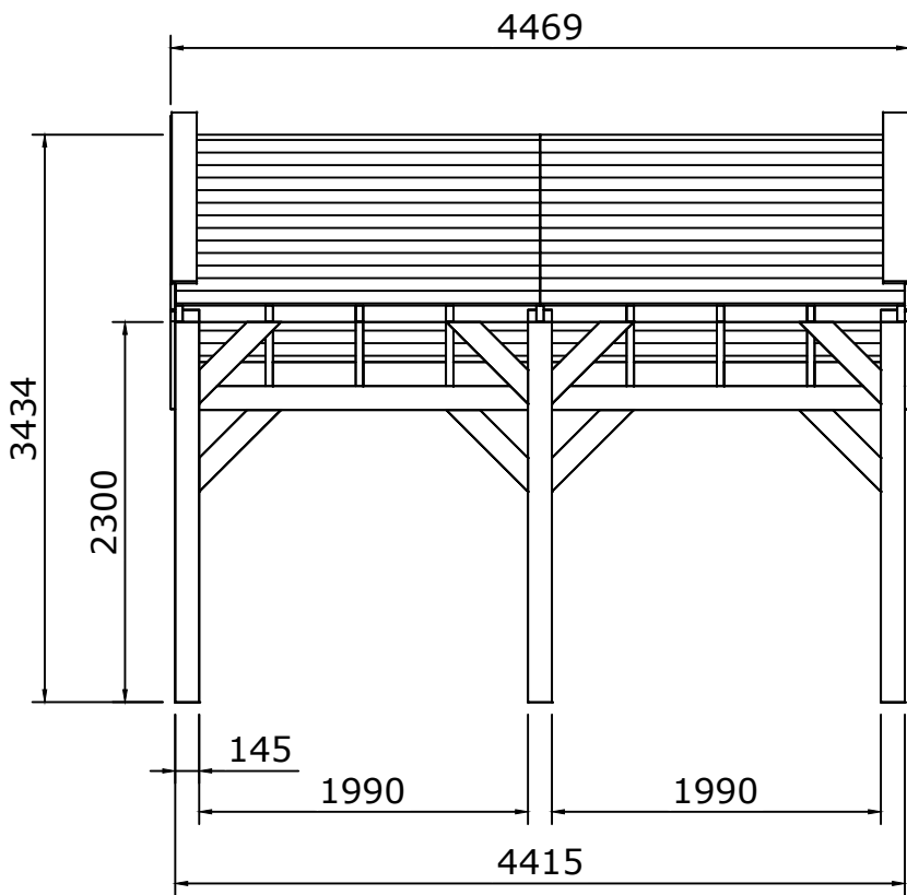
Vooraanzicht
