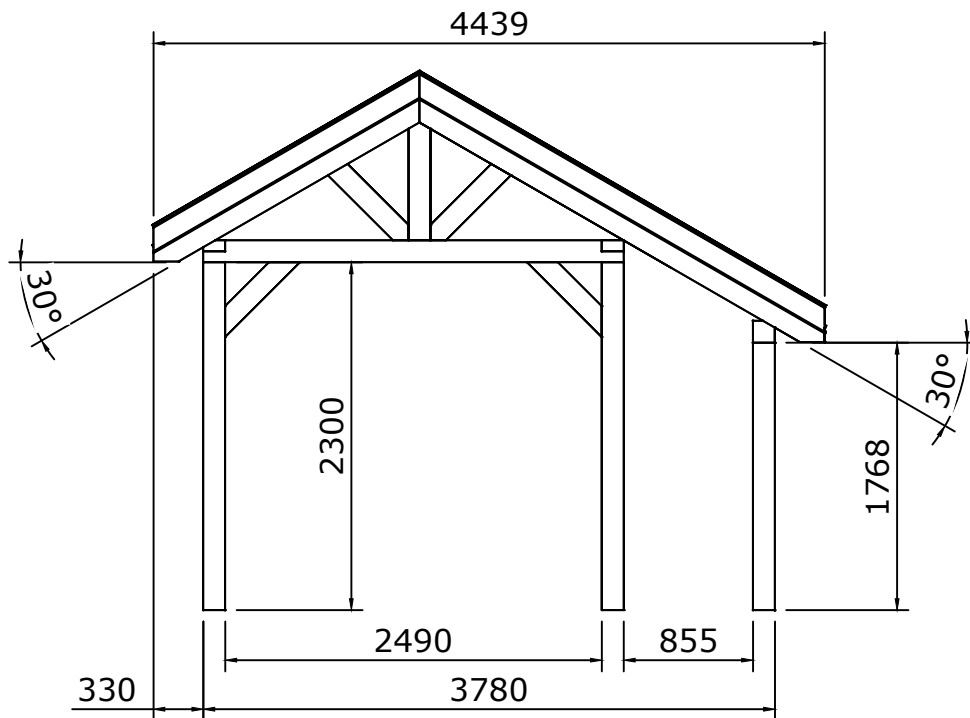
Rechter zijaanzicht
