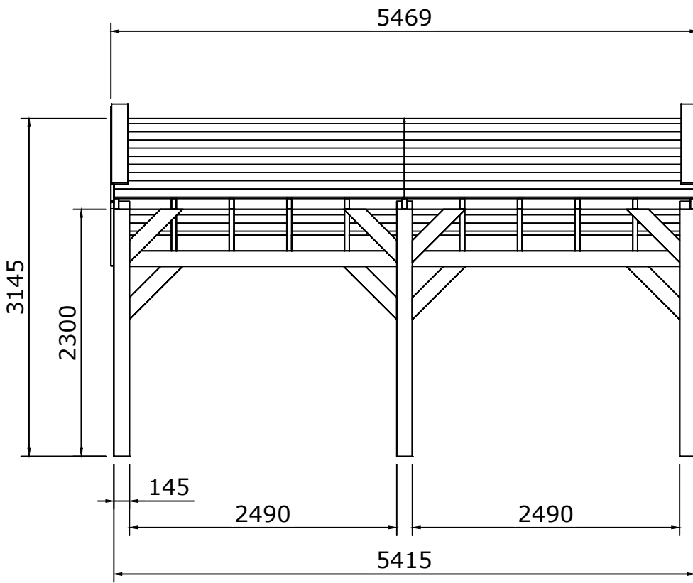
Vooraanzicht
