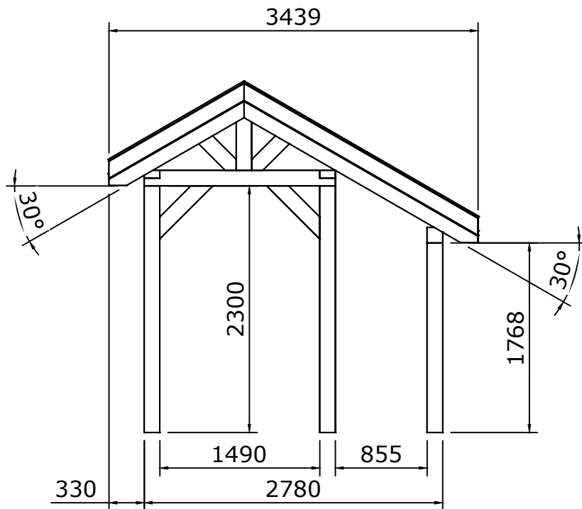
Rechter zijaanzicht
