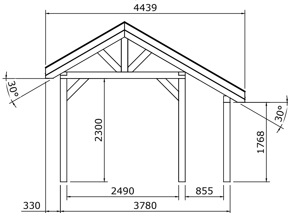
Rechter zijaanzicht
