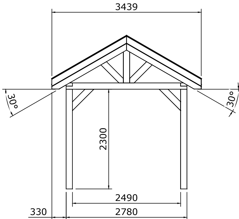
Rechter zijaanzicht
