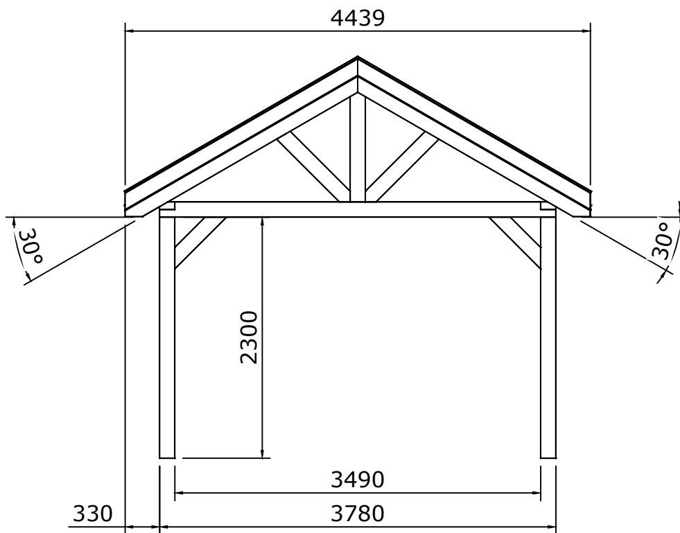
Rechter zijaanzicht
