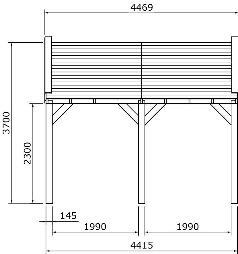
Vooraanzicht
