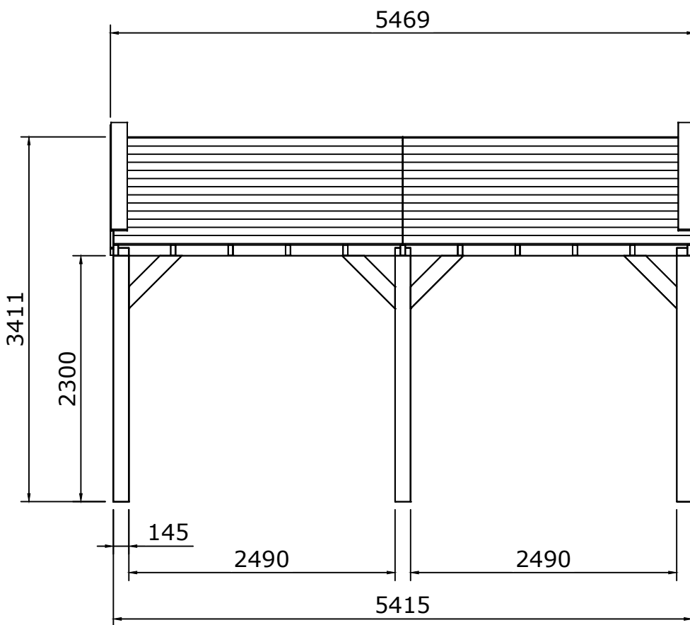
Vooraanzicht
