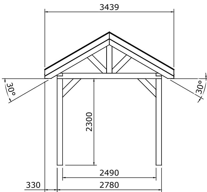
Rechter zijaanzicht
