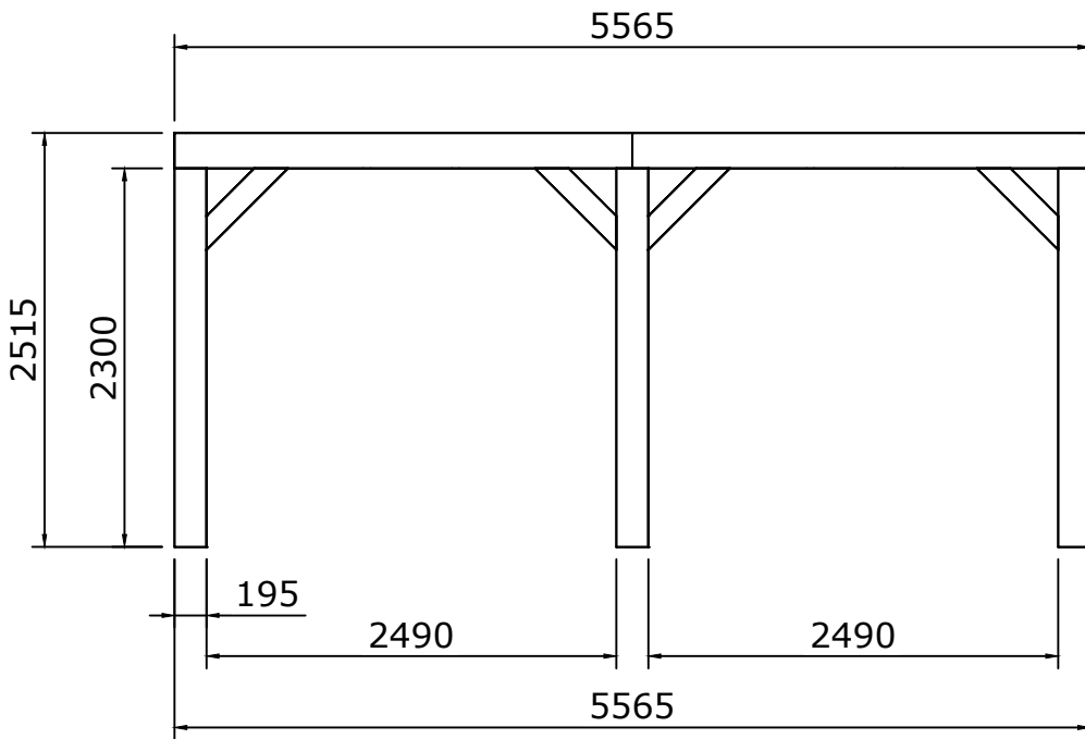
Vooraanzicht
