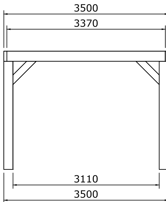
Rechter zijaanzicht
